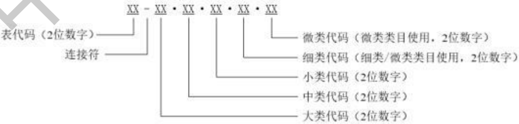
图 3 完整编码
